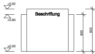
Ansicht Front
